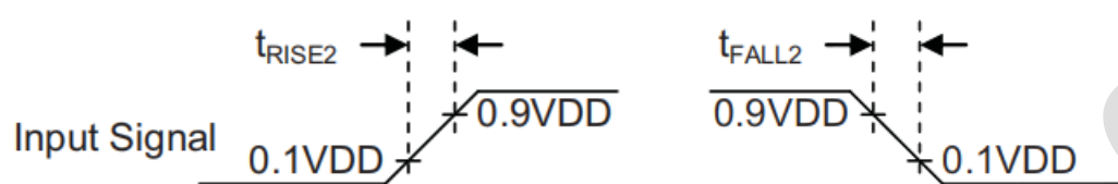
【Fig 7-2 Input Signal Rising/Falling Timing】
