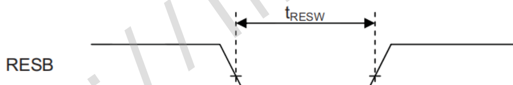
【Fig 7-3 Reset Timing Signal】
