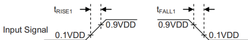
【Fig 7-1 Input Signal Rising/Falling Timing】
