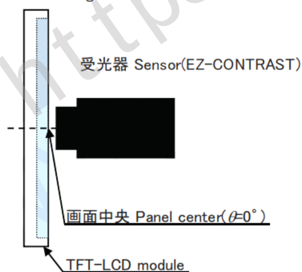
図2-1 視野角特性測定方法
