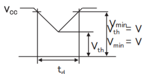
瞬時電圧降下 V CC -dip conditions
